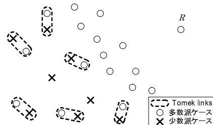
図 4 データセット C' に含まれる Tomek links Fig. 4 Tomek links in the dataset C'
